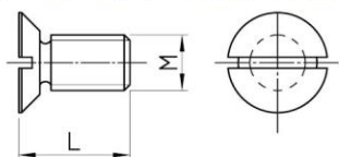
VITI TESTA SVASATA PIANA TAGLIO PER CACCIAVITE
