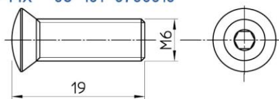
VITI NEW-FIX 08 101 0706019
