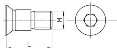
VITI SPECIALI CON ESAGONO INCASSATO
